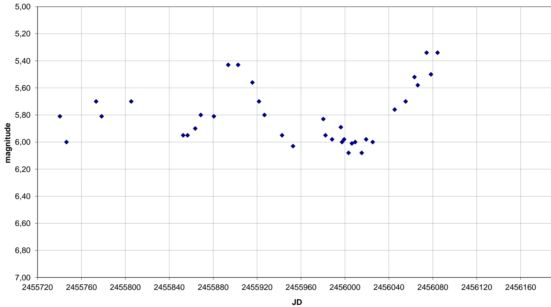
Y CVn - Grafico al 05/06/2012
