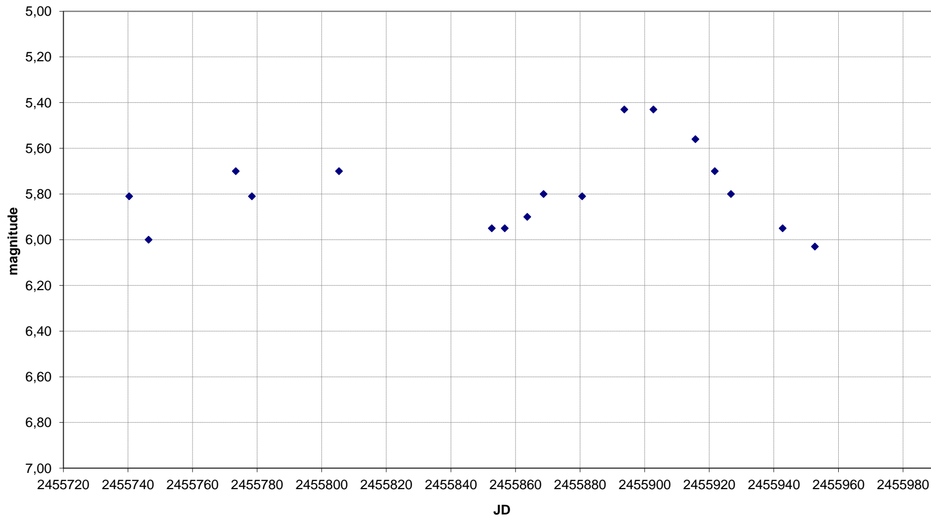
Y CVn - Grafico al 26/01/2012
