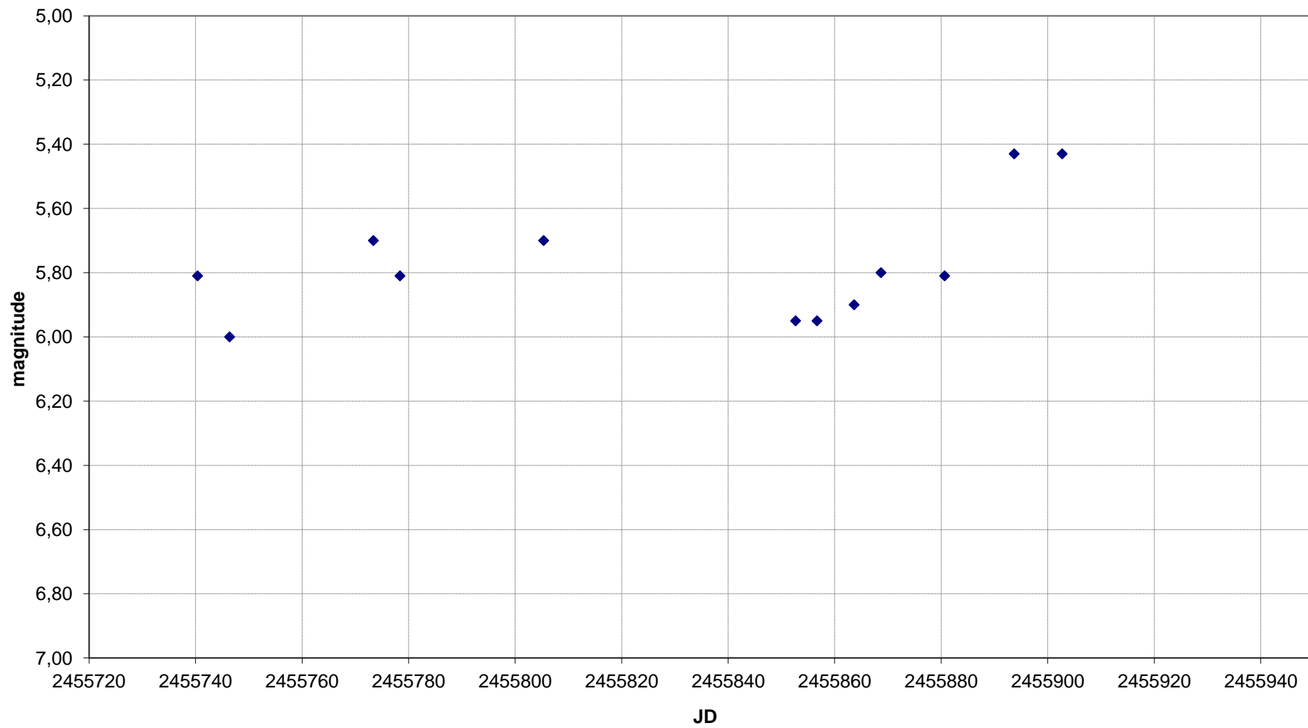
Y CVn - Grafico al 28/11/2011
