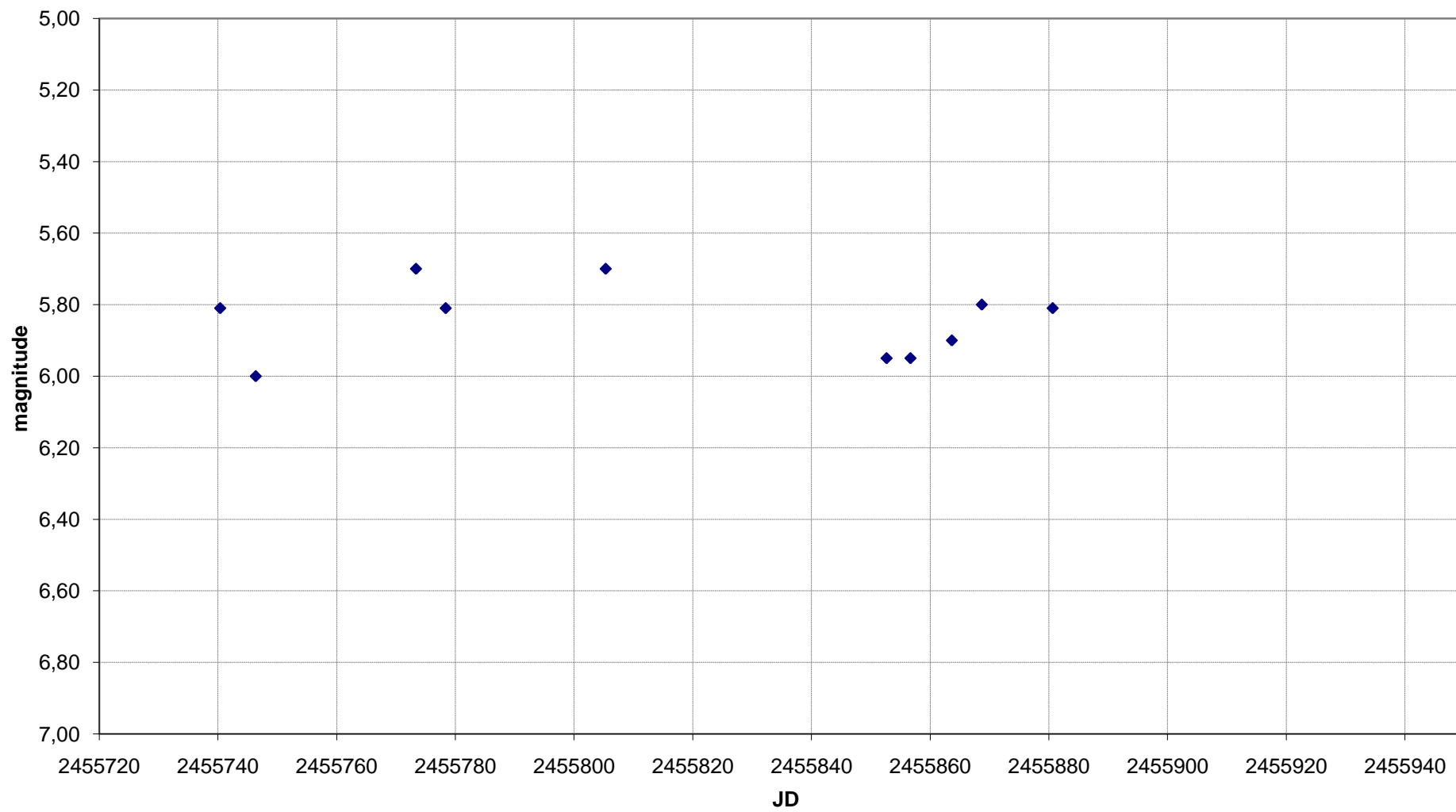
Y CVn - Grafico al 15/11/2011
