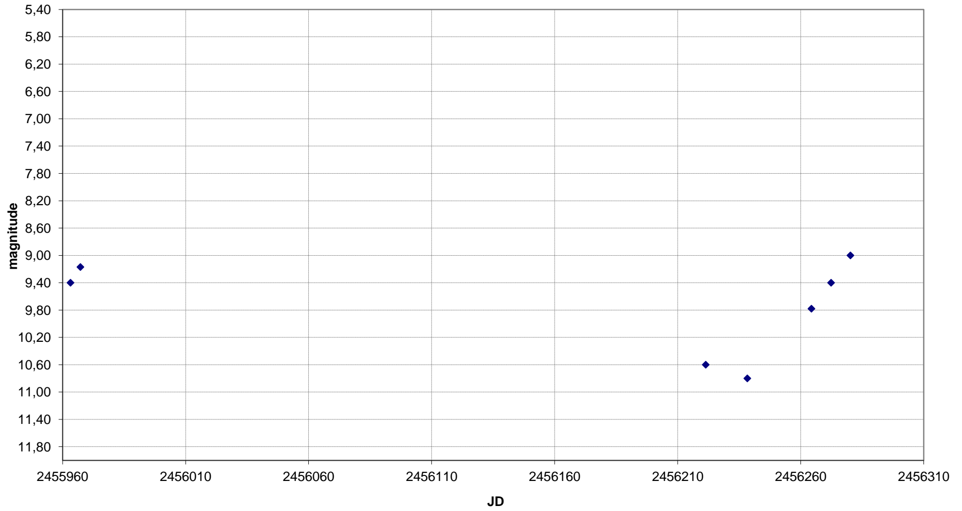
R Aqr - Grafico al 18/12/2012
