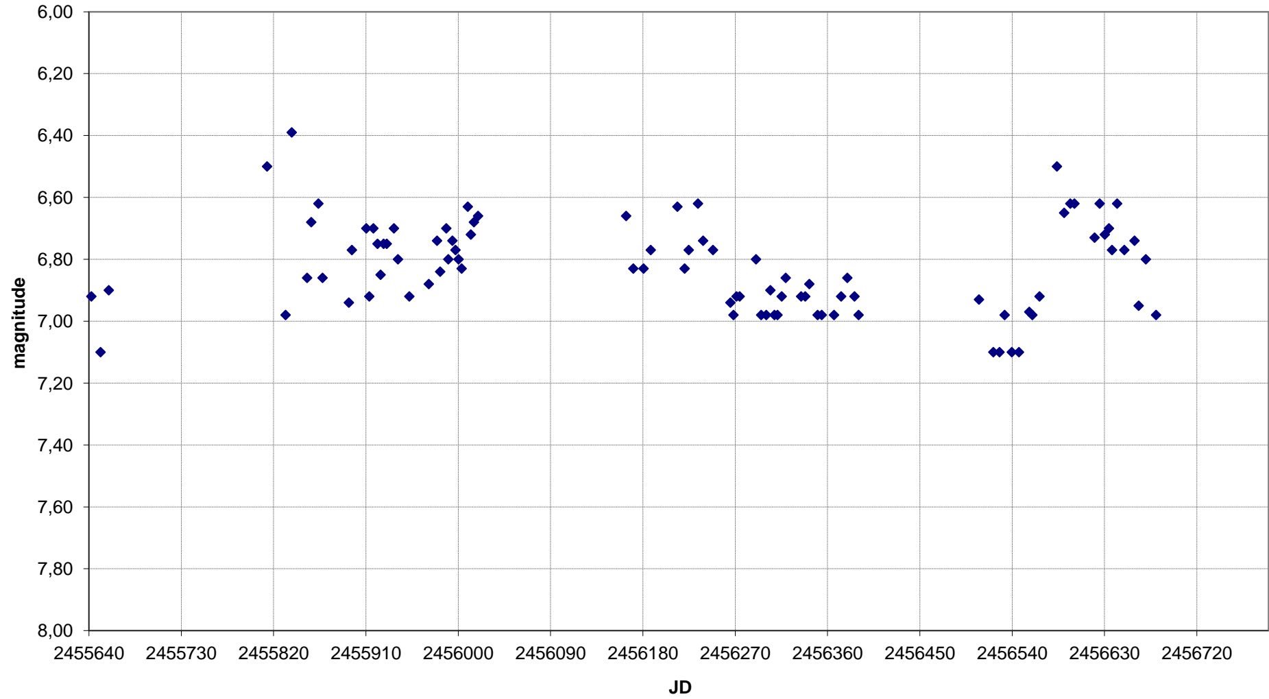
W Ori - Grafico al 22/01/2014
