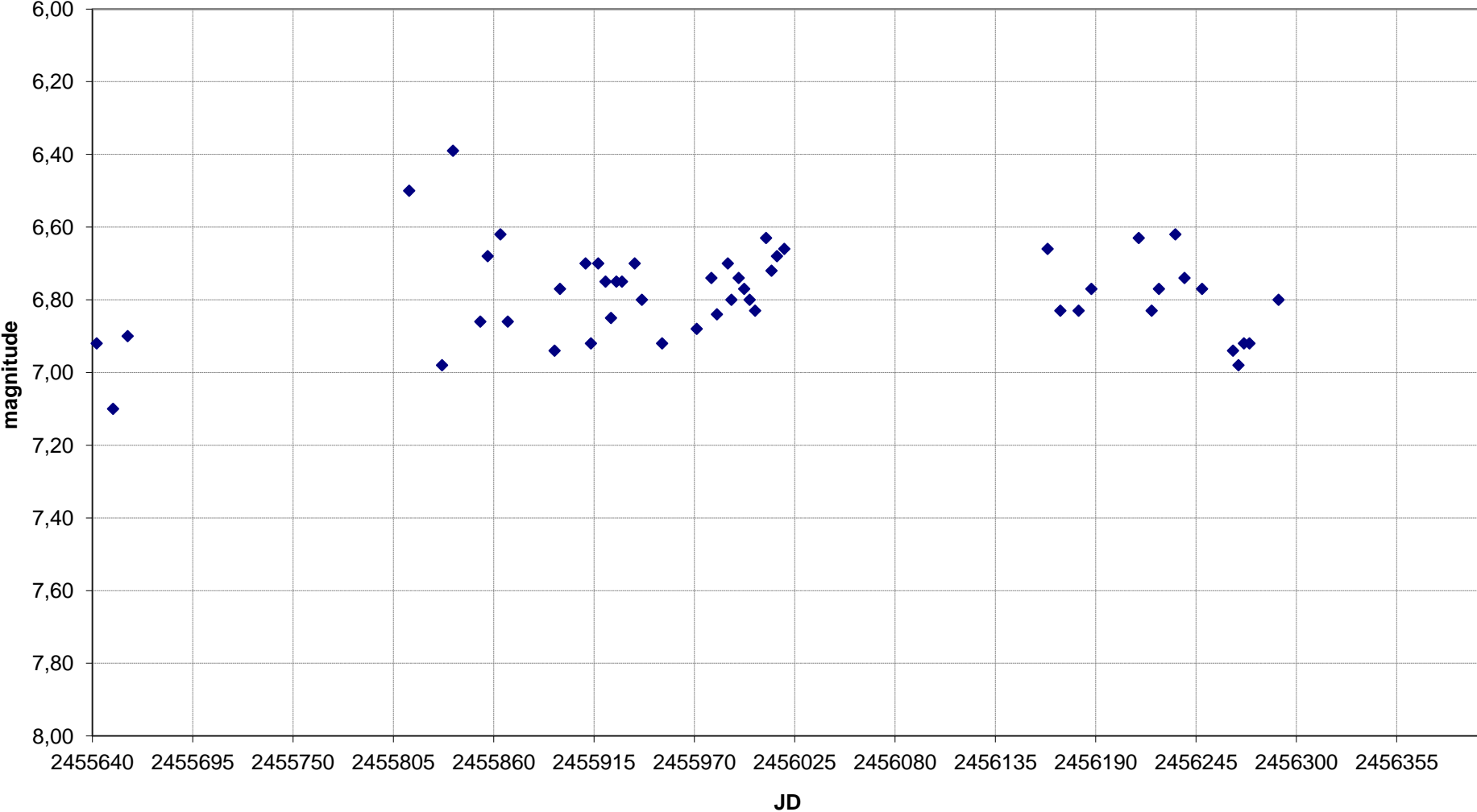
W Ori - Grafico al 28/12/2012
