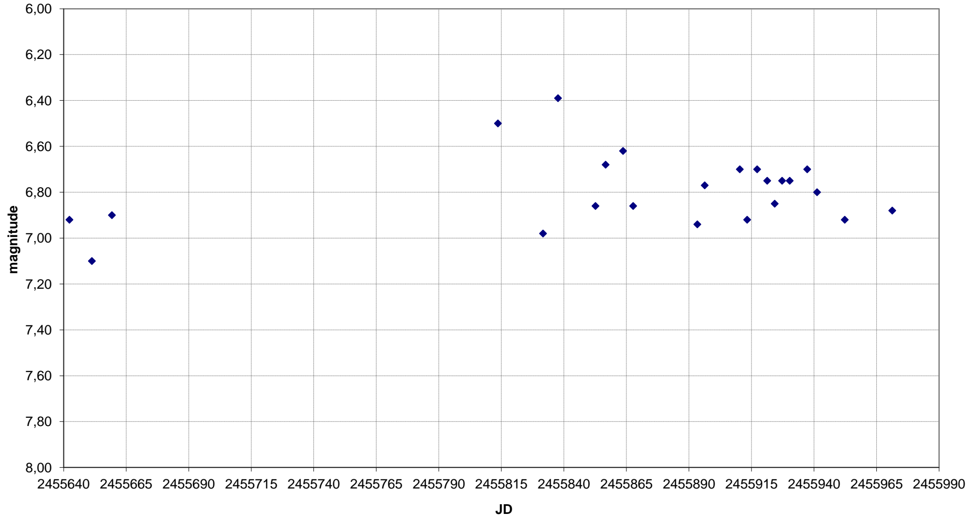
W Ori - Grafico al 13/02/2012
