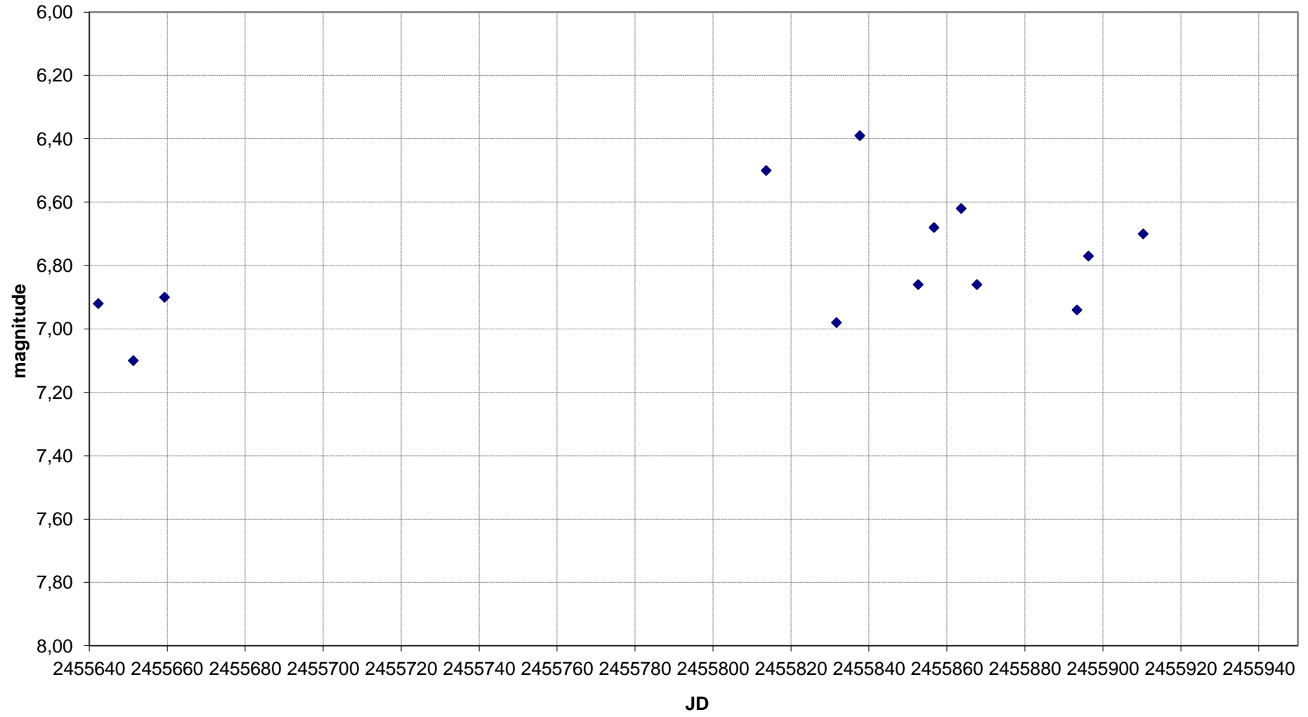
W Ori - Grafico al 14/12/2011
