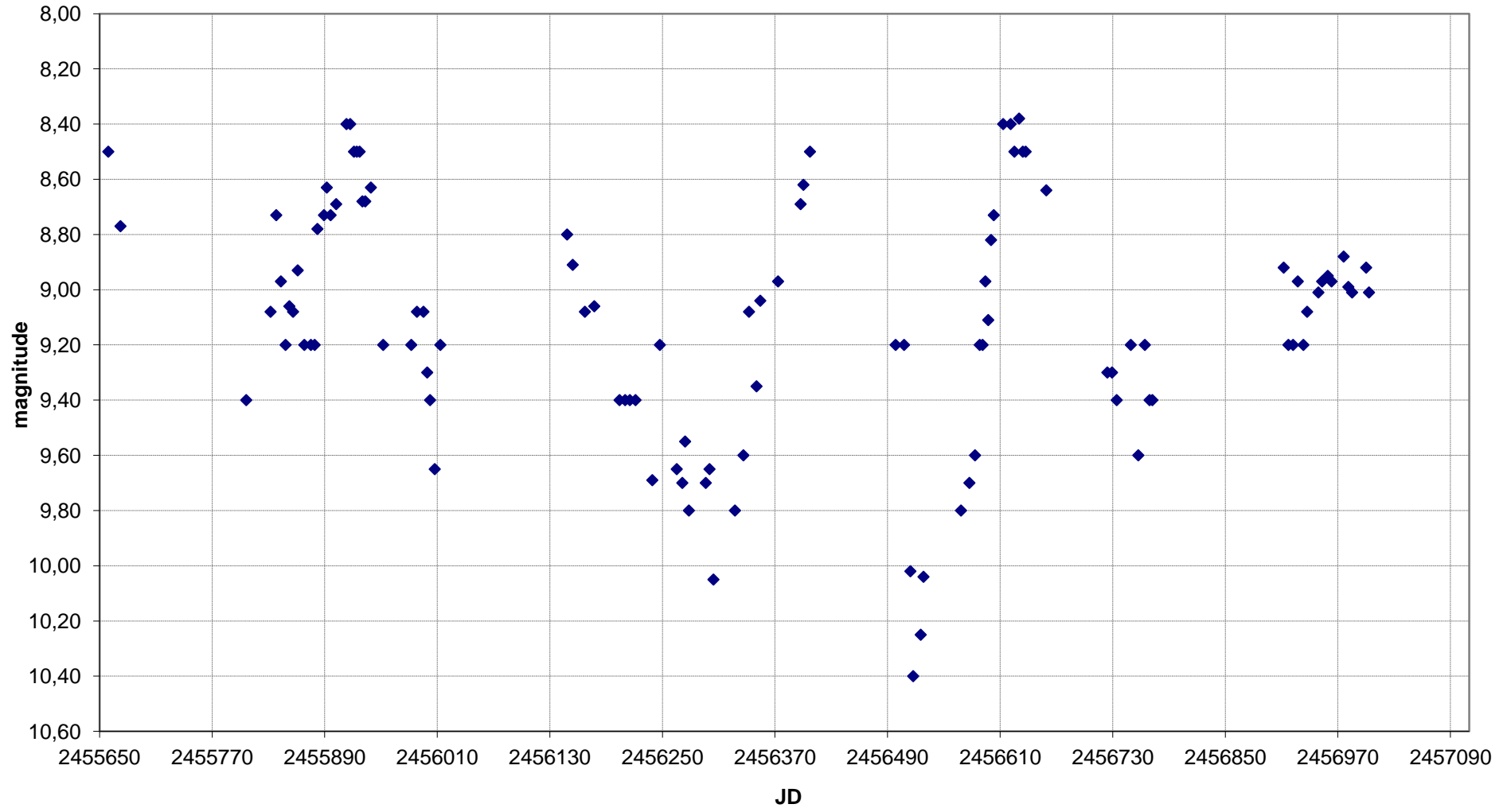
Y Per - Grafico al 11/12/2014
