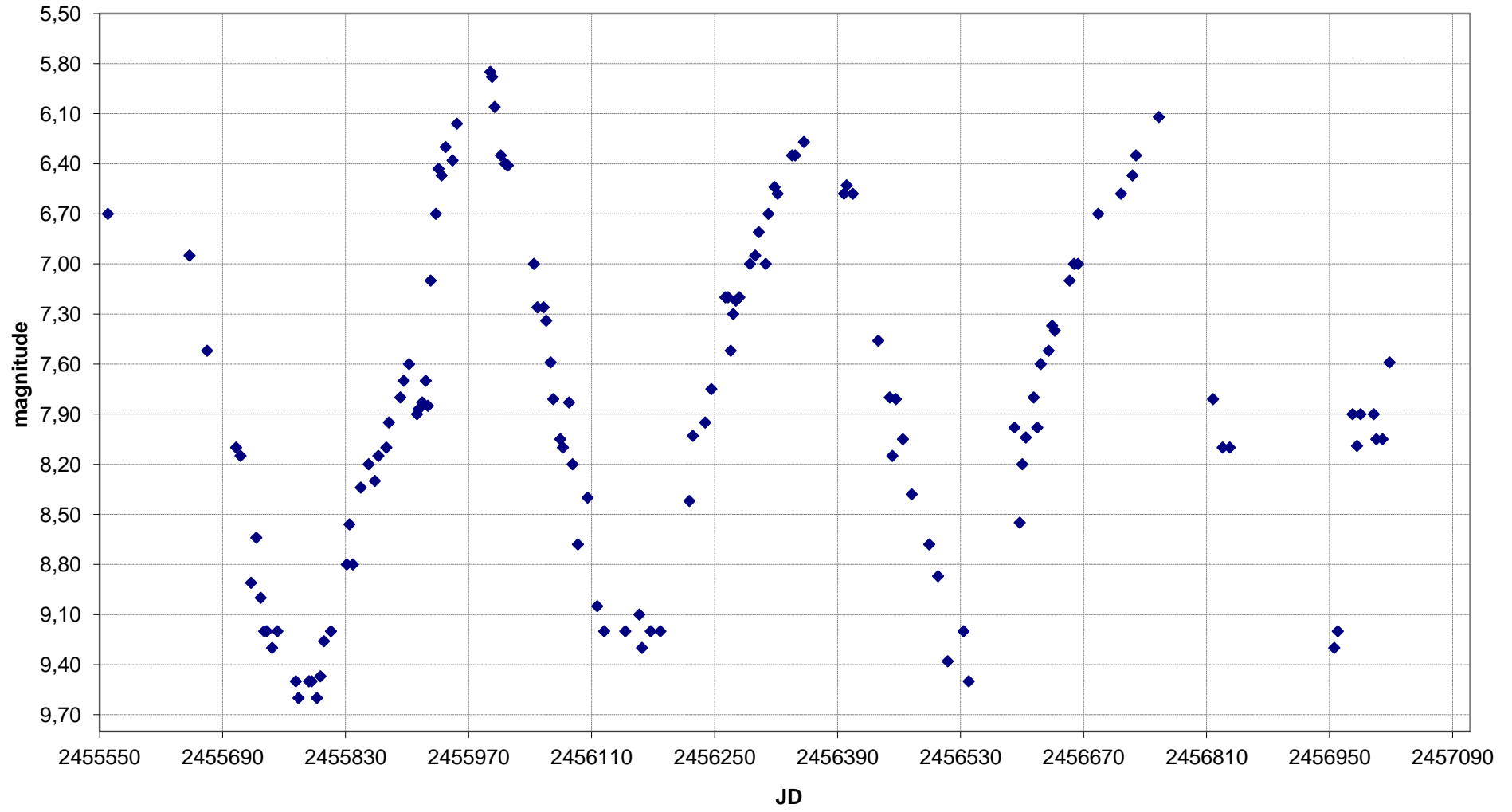
T Cep - Grafico al 26/12/2014
