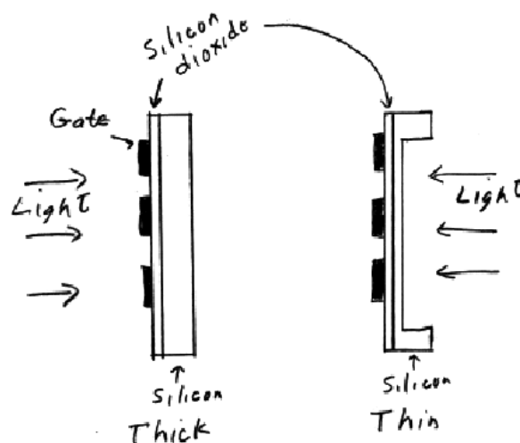
Figura 12.1. Spesso o sottile in Pizzeria? Il sensore spesso (a sinistra) ha uno strato di silicio di circa 500 micron. La luce colpisce il silicio da sinistra dopo aver passato le strutture della porta. Il sensore sottile (a destra) ha uno strato di silicio di solo circa 10 micron. La luce colpisce il sensore da destra, in tale modo non deve passare attraverso la struttura della porta.
