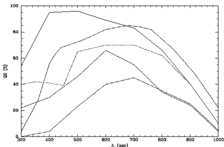
Figura 12.2. Curve di QE per cinque CCD. Dall'alto verso il basso a 500 nm: curva a tratto continuo: CCD assottigliato dell'Osservatorio Steward; curva tratto-punto: Site retro illuminato (nella camera AP7); curva punteggiata: CCD assottigliato della NRO TEK; curva tratteggiata: sensore Kodak tipo “E” (per migliorato). Questo è un sensore grosso, ma per il quale è stato utilizzato un materiale per le porte più trasparente del normale; per ultimo curva tratto-punto: vecchio sensore spesso Kodak (non E).
