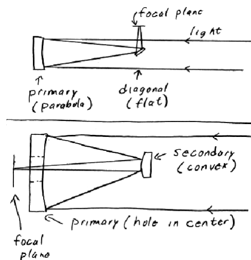
Figura 5.2. In alto: Newtoniano; in basso: sistema Cassegrain o RC. In questi sistemi lo specchio diagonale o il secondario sono di solito sostenuti da quattro sottili bracci attaccati all'interno della struttura del telescopio. Gli effetti della diffrazione della luce che passa in prossimità dei bracci sono responsabili delle familiari linee che si vedono dipartirsi dalle stelle più brillanti in molte immagini che ritraggono il cielo.
