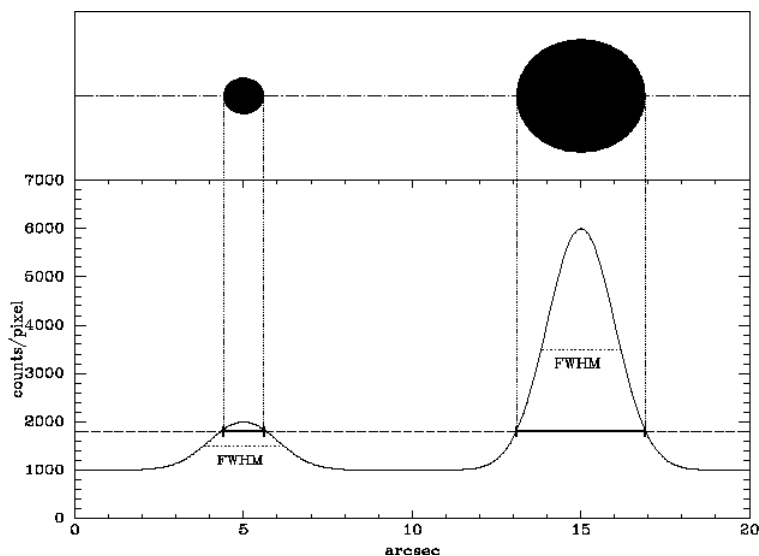
Figura 17.2. Perché le stelle brillanti appaiono più grandi di quelle deboli anche se hanno la stessa forma e dimensione dell'immagine? Riquadro in alto: Una immagine schematica di una stella brillante rispetto ad una debole (la stella brillante ha un flusso pari a 5 volte la più debole) la stella più brillante sembra più grande di quella debole. Questa immagine rappresenta tutti i pixel con valore inferiore a 1800 come “bianco” e tutti quelli con valore superiore a 1800 come “nero”. (Ignoriamo la leggera ellitticità delle stelle). Riquadro in basso: Profilo della brillantezza lungo la linea tratteggiata che attraversa i centri delle due stelle. La forma delle due stelle è esattamente la stessa, la stella brillante ha semplicemente 5 volte l'intensità luminosa sopra il fondo cielo per ogni punto rispetto la stella debole. La brillantezza lungo la linea tratteggiata al livello costante di 1800 counteggi/pixel attraverso l'immagine mostra che, mentre le stelle brillante e debole hanno la stessa forma (stessa PSF) la stella più luminosa sembra più grande per ogni livello di grigio sull'immagine. Le linee punteggiate sui profili stellari indicano la FWHM per ogni stella (qui la FWHM è circa 2,3 arcsec). La linea continua che interseca i profili al valore counteggi/pixel=1800 dà le dimensioni della stella sull'immagine nel riquadro superiore. Notare: in una immagine CCD ed in un grafico reali dovremmo essere in grado di vedere i singoli pixel così che il bordo dell'immagine CCD della stella dovrebbe essere costituito da un insieme di quadrati e il profilo dell'intensità lungo una singola linea dovrebbe sembrare un insieme di gradini costituiti da pixel singoli.
