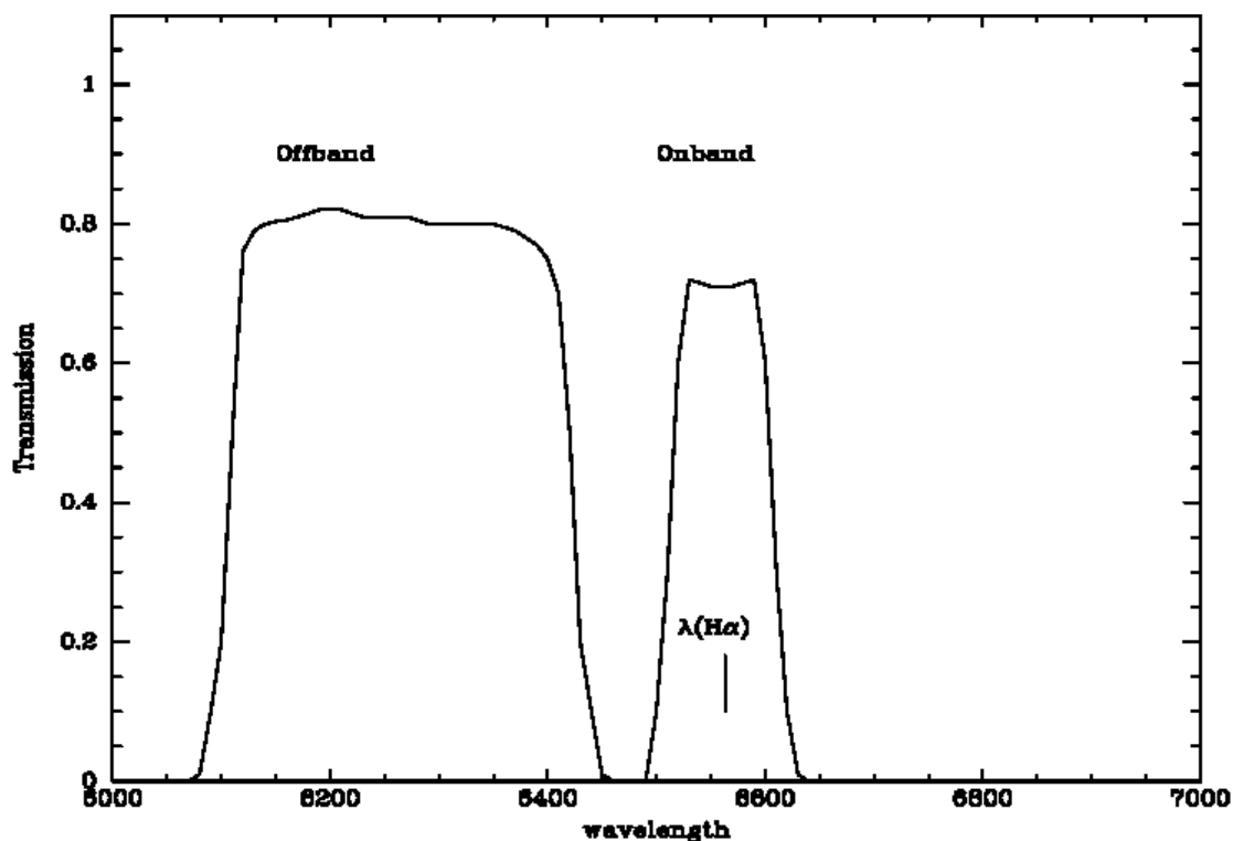
Figura 22.2. Bande passanti di un tipico set di filtri impiegati per riprendere immagini nella riga H_\alpha . Il filtro passante (onband) trasmette la radiazione H_\alpha e quella del continuo, mentre il filtro di arresto (offband) lascia passare solo la radiazione dello spettro continuo in prossimità della linea H_\alpha . Quando si osservano galassie esterne, si utilizza, per galassie in diversi intervalli di redshift, un insieme di filtri onband con diverse lunghezze d'onda centrali, in quanto la lunghezza d'onda della linea di emissione H_\alpha è diversa in funzione del redshift.
