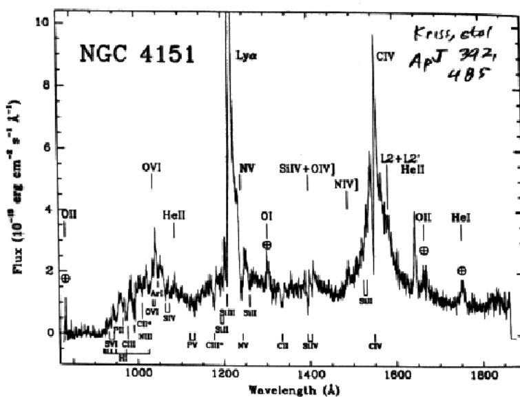
Figura 3.1. Esempio di spettro di un oggetto astronomico, il nucleo attivo nella galassia NGC 4151. Notare le unità sull'asse y ( 10^{-13} \text{ erg s}^{-1} \text{ cm}^{-2} \text{ \AA}^{-1} ). Si noti il range di unità sull'asse x – questo spettro non è stato ovviamente registrato con un telescopio basato a terra!
