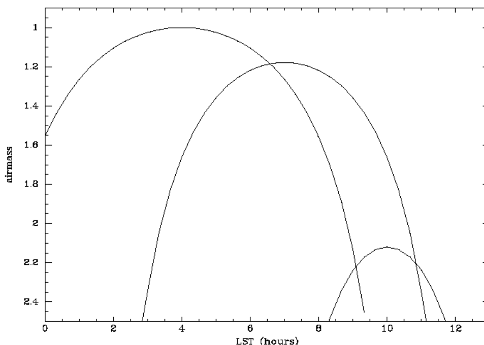
Figura 25.3. Esempio di airmass in funzione del tempo per osservazioni da Kitt Peak (lat =32°). Il primo oggetto ha una declinazione di 32 gradi, cosicché transita allo zenit ad airmass=1. L'oggetto successivo transita 32 gradi a sud dello zenit (come un campo Landolt sull'equatore, dec=0°). Il terzo oggetto è ad una declinazione di -30°, molto vicina all'orizzonte di Kitt Peak, tanto che esso non supera mai il valore 2,1 di airmass.
