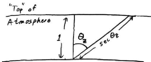
Figura 9.4. La massa d'aria è uguale alla secante dell'angolo zenitale, tranne che in prossimità dell'orizzonte, dove si deve considerare la curvatura dell'atmosfera.
