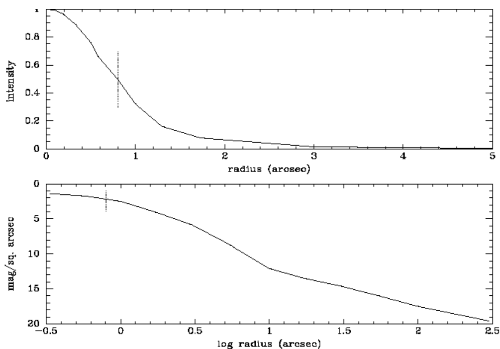
Figura 17.1. Tipica funzione “Point Spread Function” (PSF). Questa particolare PSF appartiene ad una stella vista attraverso un seeing pari a 1,6 arcsec FWHM (King PASP 83,199, 1971). Riquadro in alto: Intensità radiale della luce (normalizzata al centro =1,0) della PSF sopra descritta. Su questo grafico il valore HWHM, il raggio al quale la PSF scende a metà del valore centrale di picco, è indicata tramite una linea tratteggiata verticale. Riquadro in basso: E’ riportato nel grafico l’andamento della brillantezza superficiale (mag/arcsec 2 ) (essenzialmente il logaritmo dell’intensità) rispetto al logaritmo del raggio dal centro dell’immagine. La HWHM è nuovamente indicata da una linea tratteggiata verticale. Notare che il riquadro in basso mostra la PSF sino ad un grande valore del raggio (oltre i 300 arcsec) rispetto a quello mostrato nel riquadro superiore (5 arcsec). L’asse y logaritmico permette di vedere le regioni molto deboli della PSF sino ad un grande raggio invisibile nel riquadro superiore in cui l’asse y è lineare. Notare che la PSF decade semplicemente – non c’è confine oltre il quale la PSF raggiunge il valore zero.
