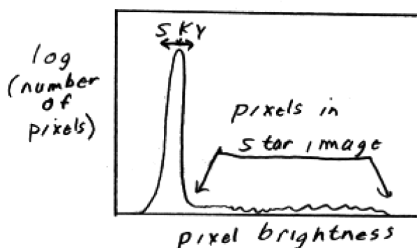
Figura 15.1. Istogramma di un campo stellare sparso. Poiché le immagini stellari coprono una grande gamma di intensità di pixel, ma una piccola parte dell'area dell'immagine, i pixel delle stelle sono pochi di numero ma spaziano in una vasta gamma di luminosità.
