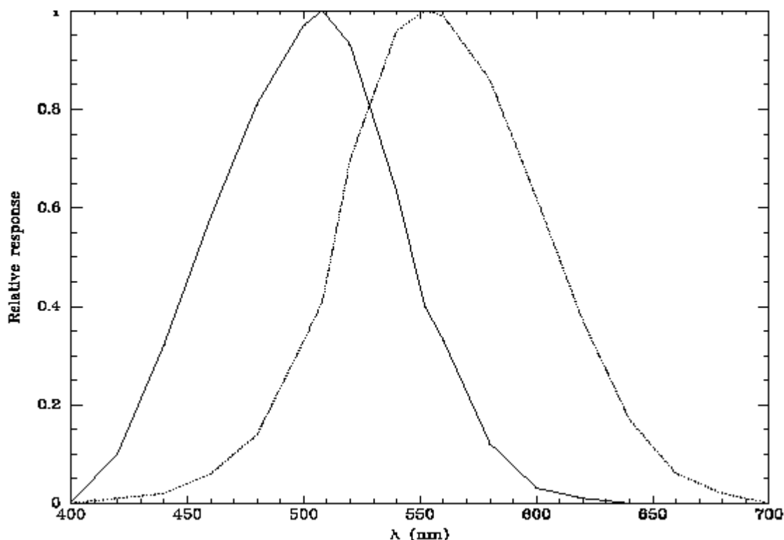
Figura 11.1. Sensibilità nelle bande d'onda dell'occhio umano. La linea continua rappresenta la visione scotopica, quella tratteggiata la fotopica. L'asse delle y non è calibrato in termini di unità reali; è una risposta relativa al picco.
