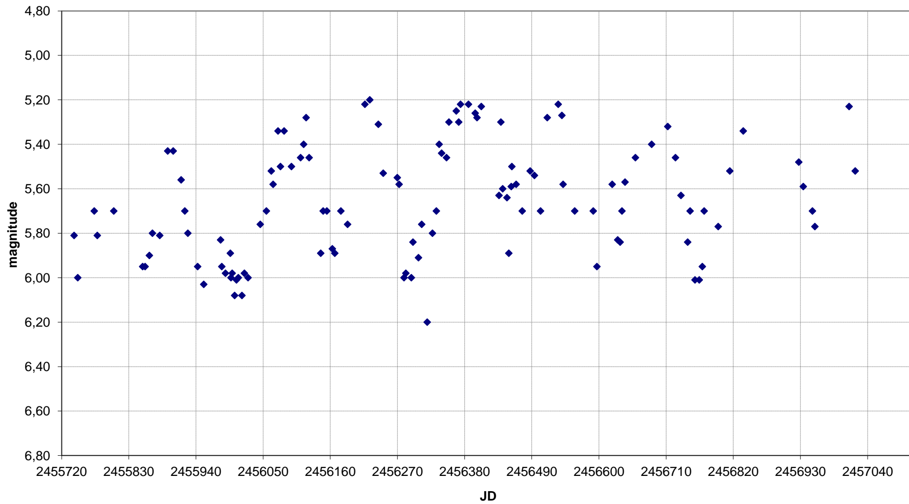
Y CVn - Grafico al 18/12/2014
