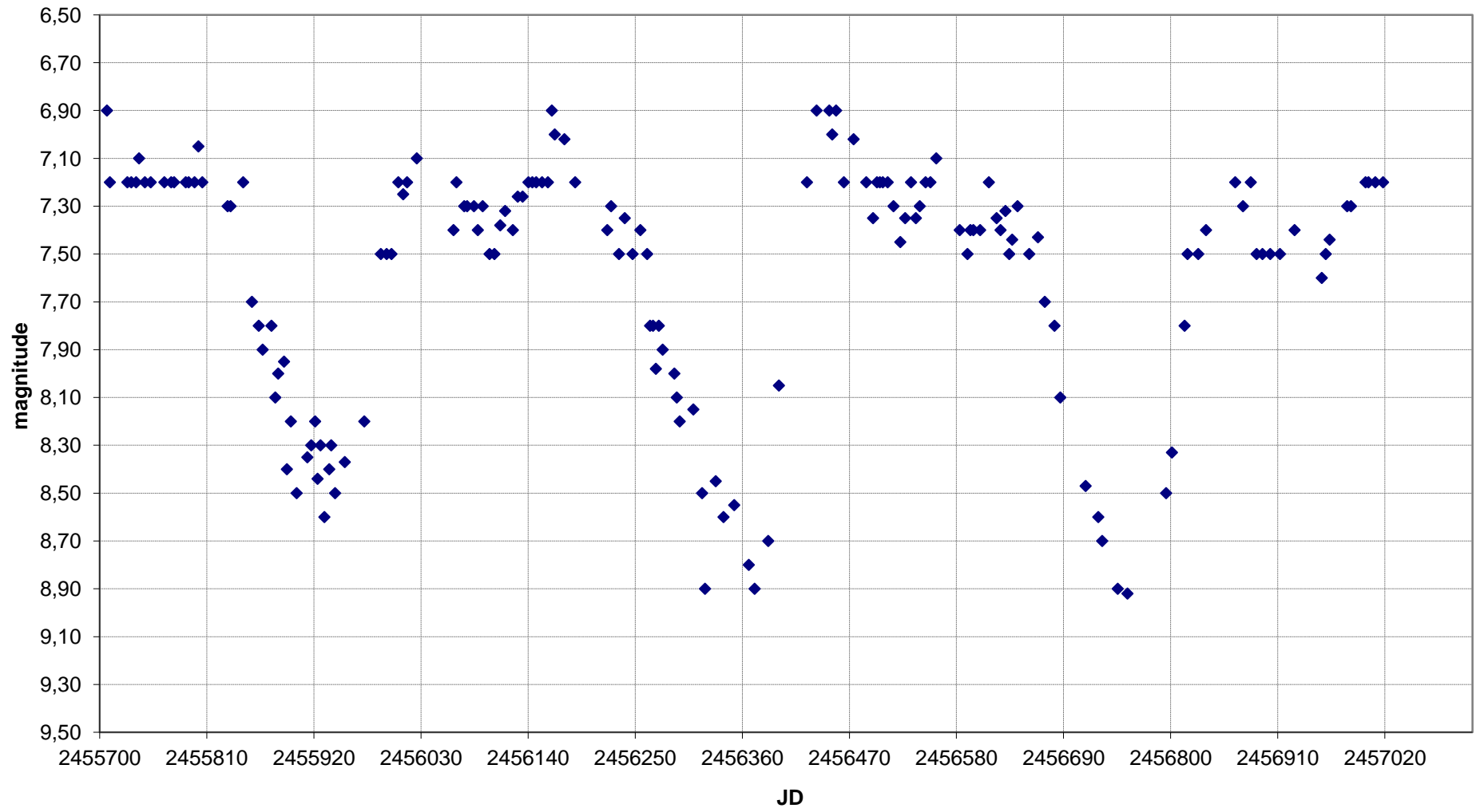
RS Cyg - Grafico al 26/12/2014
